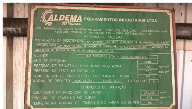
Boiler nº 1
